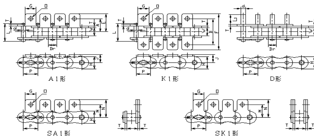
チェーン各部寸法
